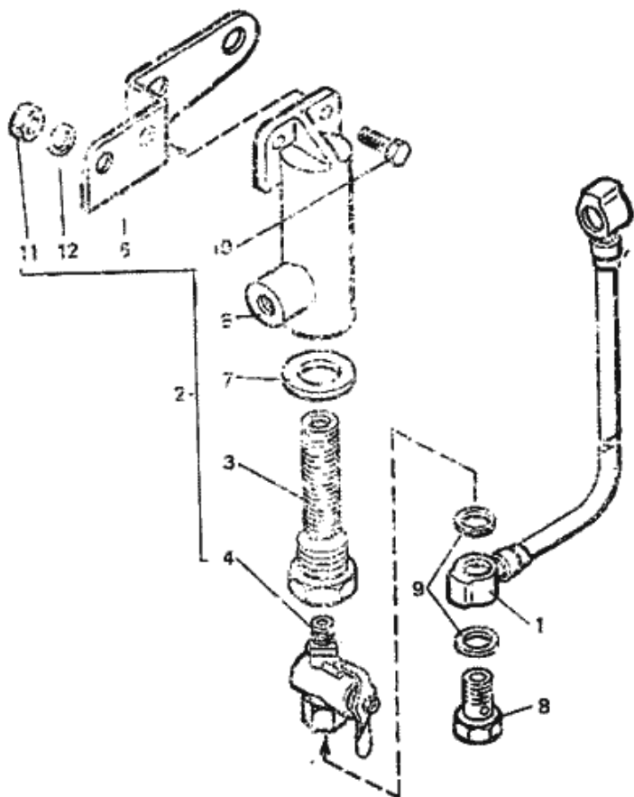
Рис. 68. Фильтр-отстойник Т40АН-1105080
